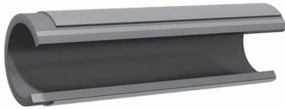
Трубы из ПЭ 100, ПЭ 100+, ПЭ 100 RC с защитной оболочкой (PS) диаметром от 63 до 1200 мм
