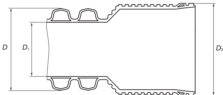
Рис. 1.2. Труба SUNSET с раструбом исп. 2 (с уменьшенной высотой гофра в месте соединения с раструбом)
